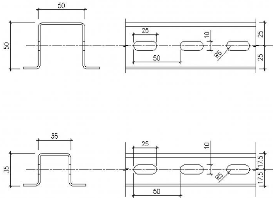
Рис.6 Схема перфорации омега-профиля
